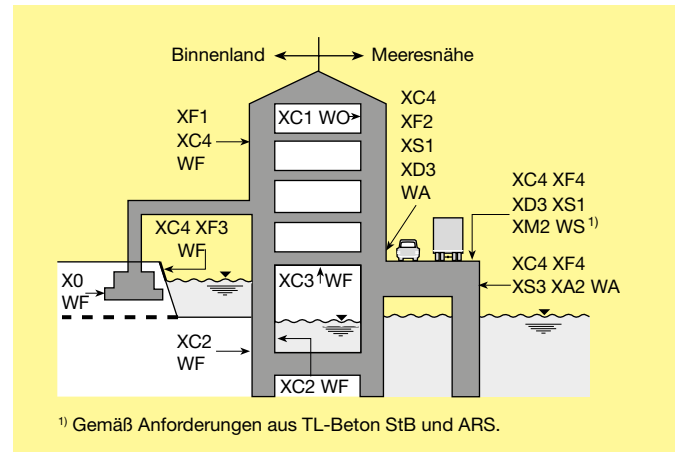
Bild 2: Beispiele für mehrere, gleichzeitig zutreffende Expositions- und Feuchtigkeitsklassen im Hoch- und Ingenieurbau in Anlehnung an [3]
