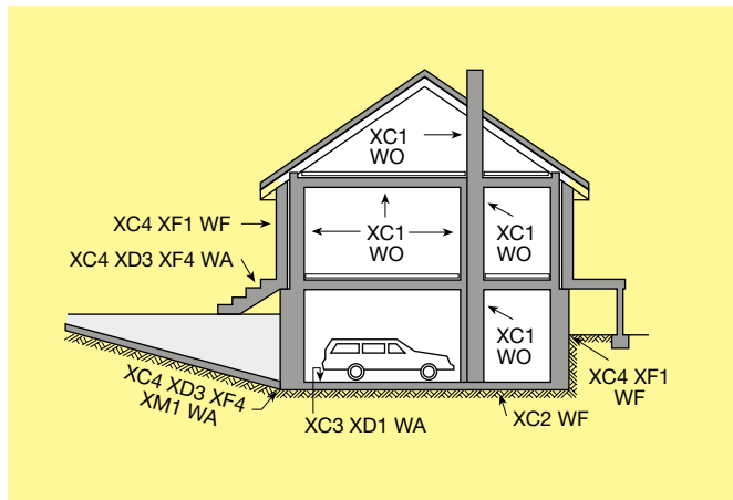
Bild 1: Beispiele für mehrere, gleichzeitig zutreffende Expositions- und Feuchtigkeitsklassen an einem Wohnhaus
